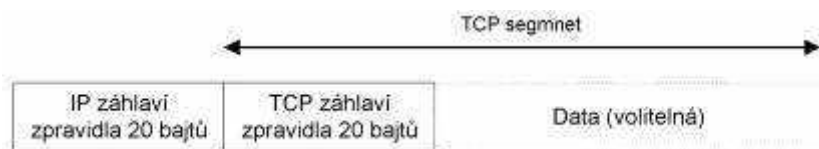
Obr. 21 TCP segment; zdroj: (4)
